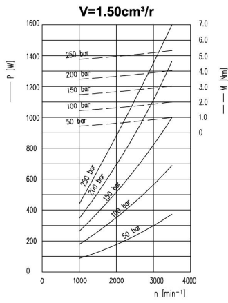
0.5系列功率性能曲线表/Group 0.5 Power Performance Curve Table
