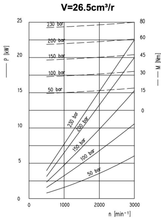
2.5系列功率性能曲线表/Group 2.5 Power Performance Curve Table
