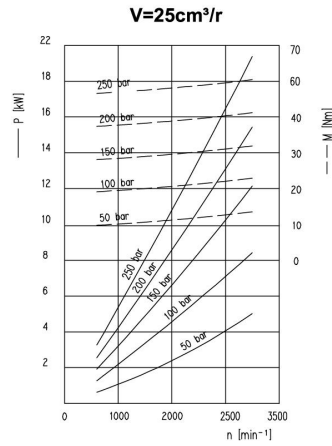
2.5D系列功率性能曲线表/Group 2.5D Power Performance Curve Table
